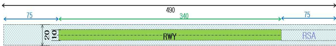
[그림 3] 활주로 양쪽에 안전구역을 설치한 활주로 평면도
